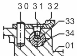
DETALHE E FIXAÇÃO DA TRAVA
